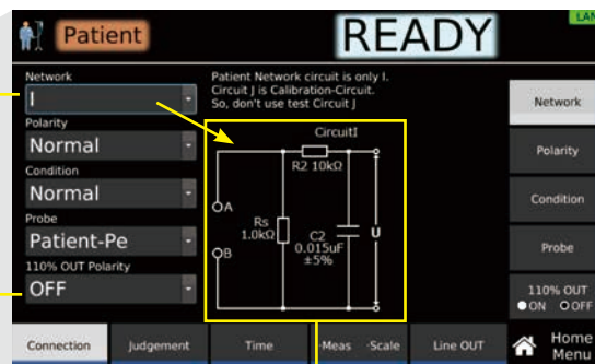
Messstromkreis-Netzwerk (Netzwerk I IEC60601-1)
