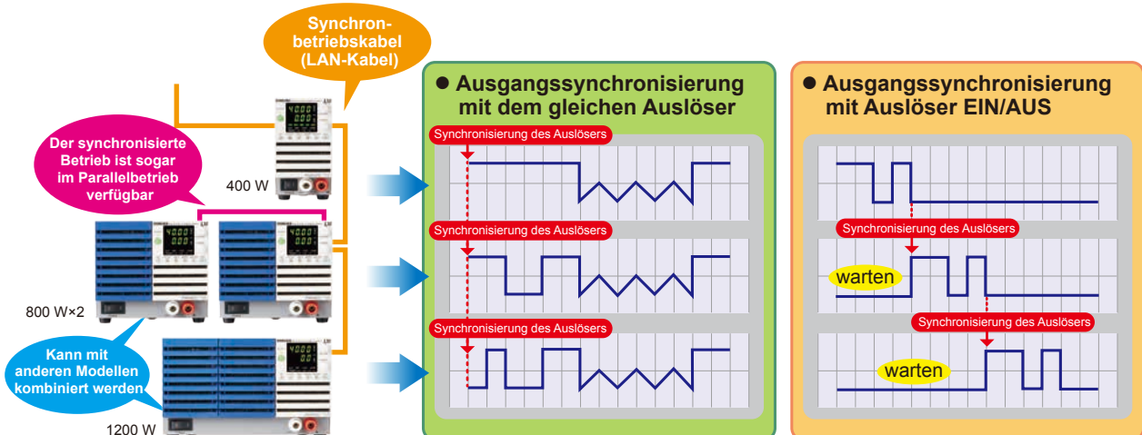
Die Ausgangsänderungen können mit demselben Auslösersignal synchronisiert werden.
